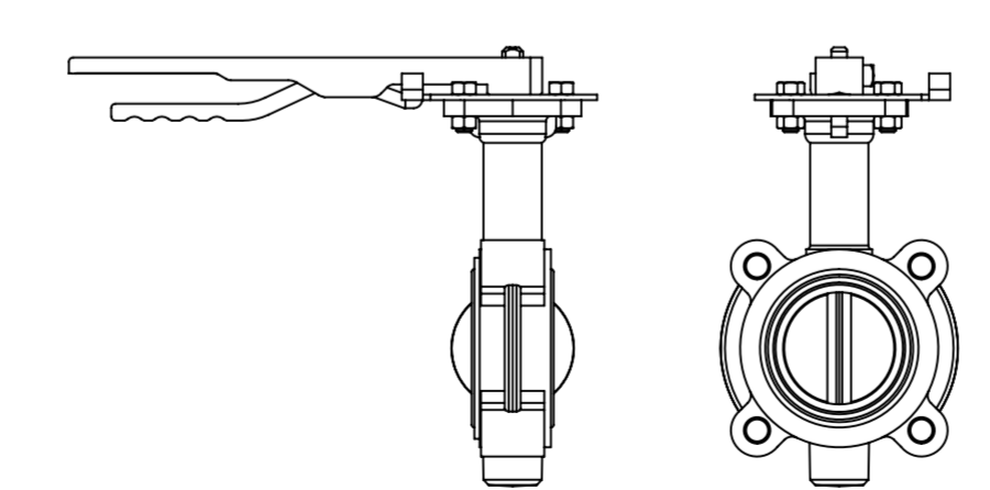
Läppäventtiili
